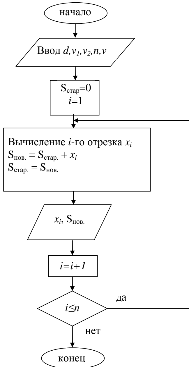
Рис. 1.4. Третий вариант алгоритма
