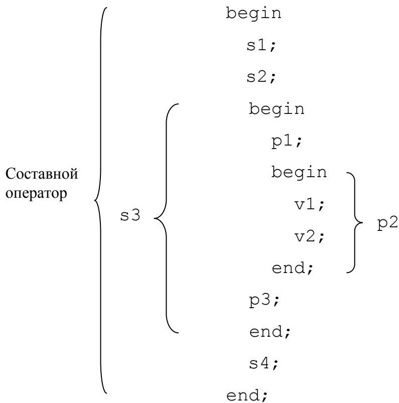
Рис. 2.53. Вложенные составные операторы
