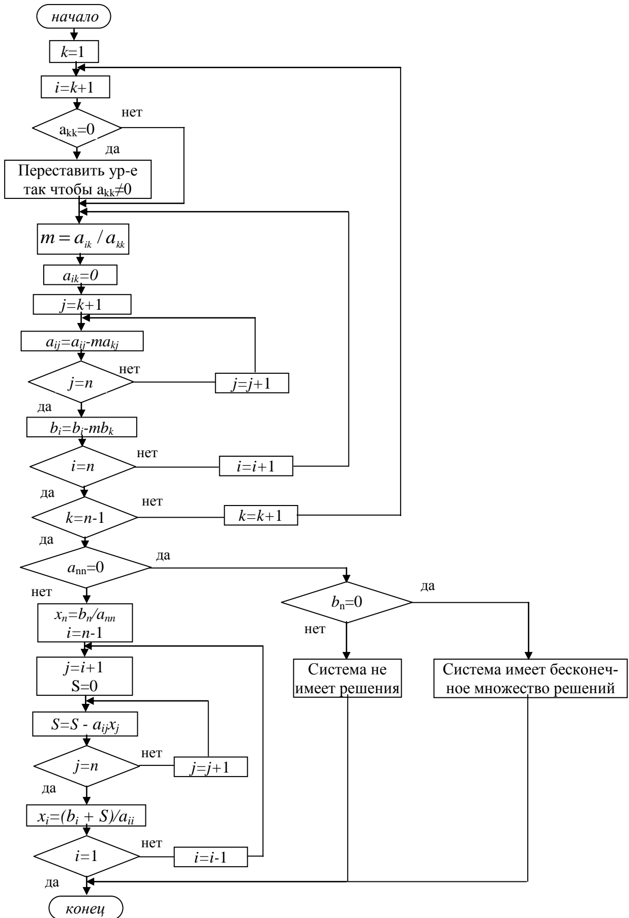
Рис. 1.12. Алгоритм Гаусса
