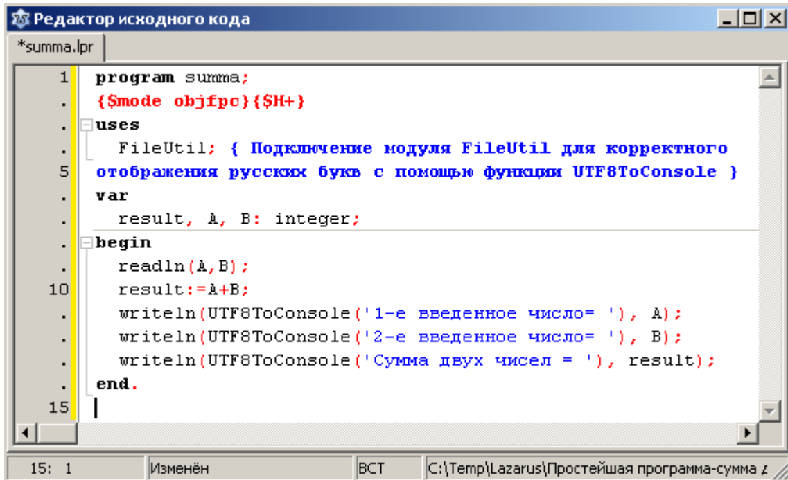
Рис. 2.22. Окно редактора исходного кода в Windows
