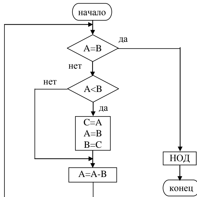
Рис. 1.1. Алгоритм Евклида
