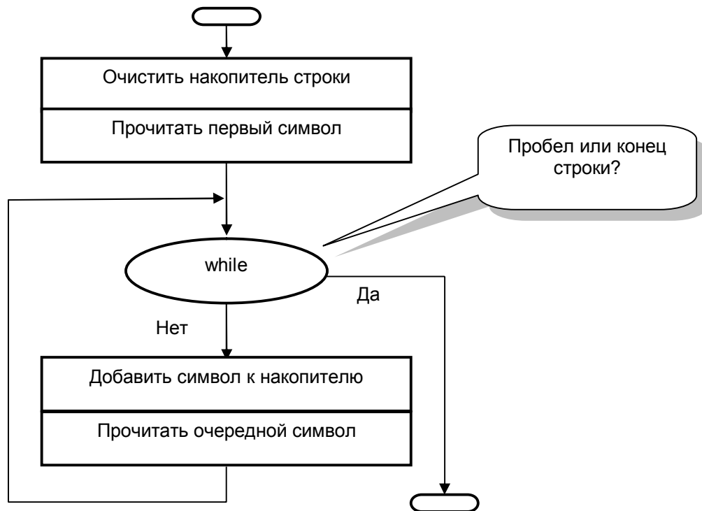
Рис. 71 – Упрощенный алгоритм побуквенного чтения фамилии
