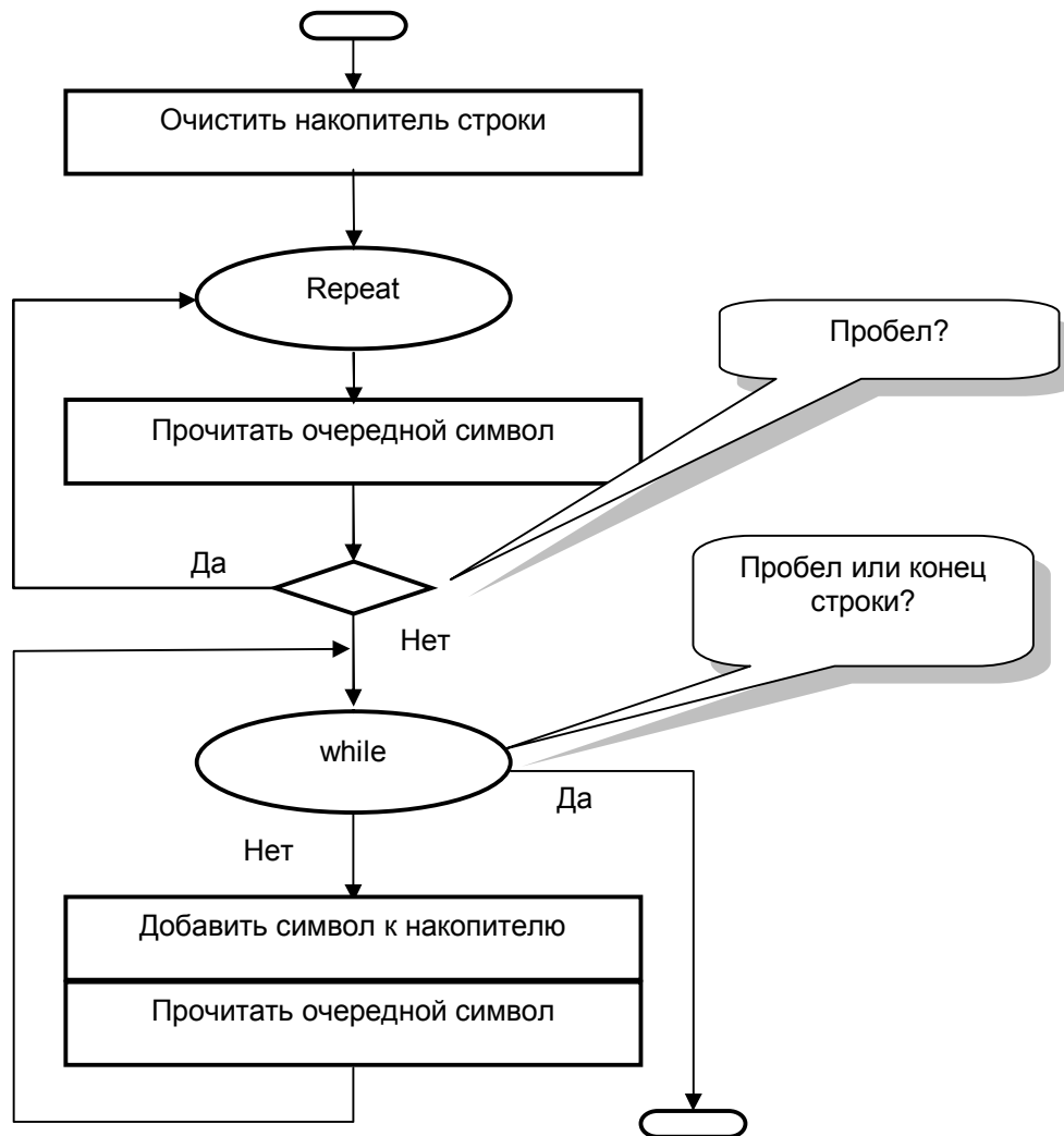
Рис. 72 – Усовершенствованный алгоритм побуквенного чтения фамилии
