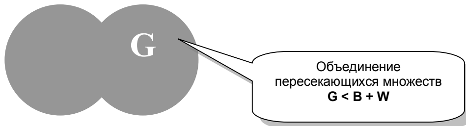
Рис. 82 – Объединение пересекающихся множеств G < B + W
