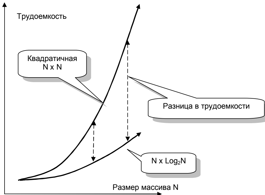
Рис. 97 – Рост трудоемкости сортировки с ростом размера массива
