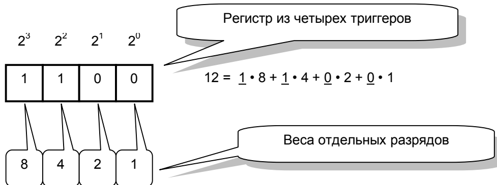
Рис. 106 – Изображение числа 12 в двоичной системе
