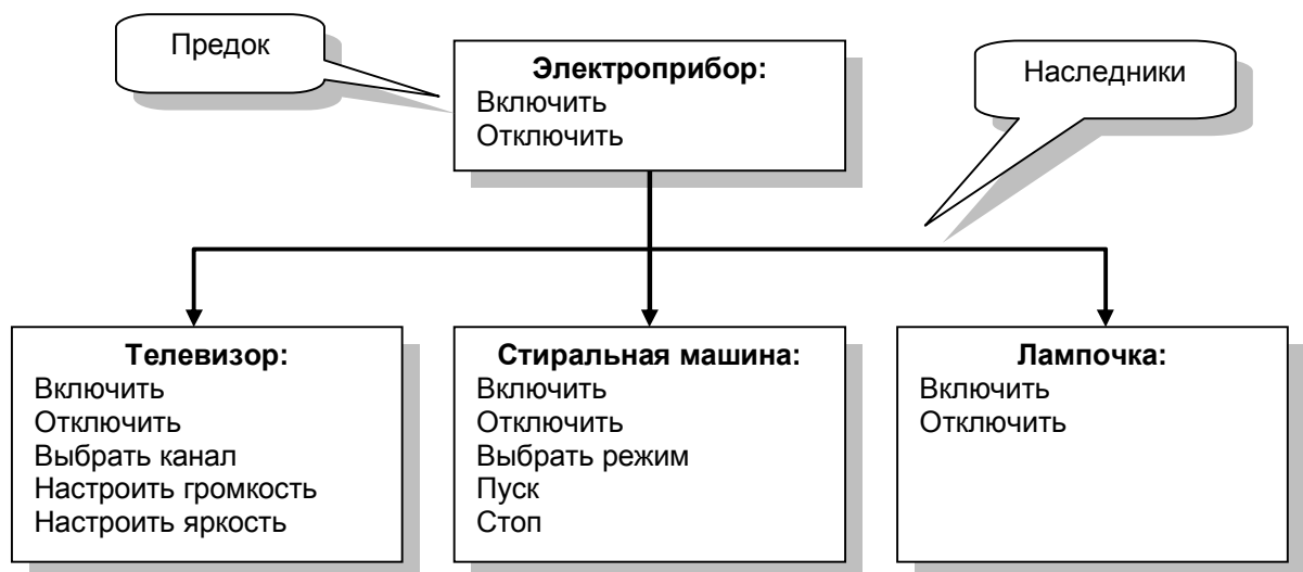
Рис. 153 – Иерархия электрических приборов
